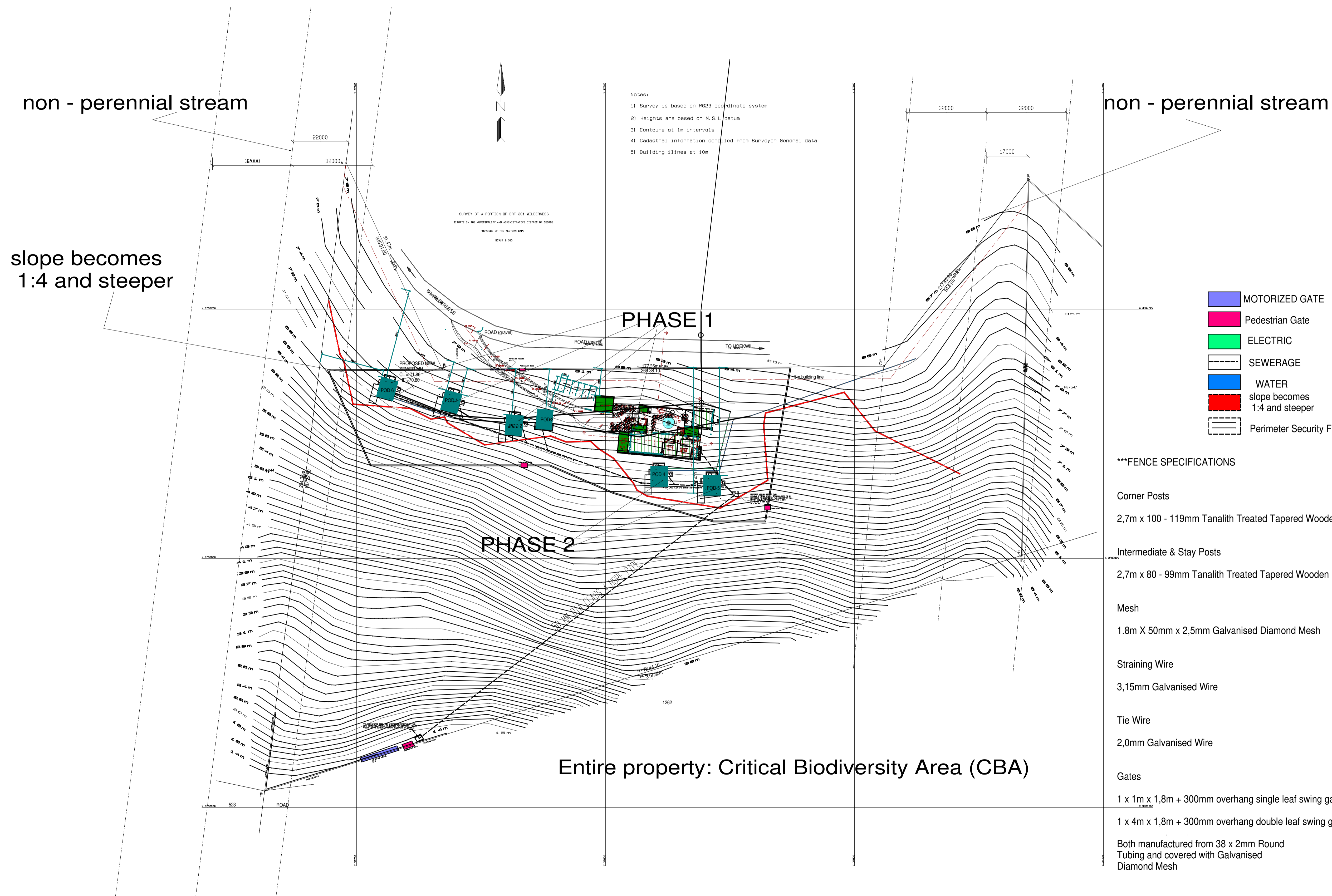
SITEPLAN 1:800
